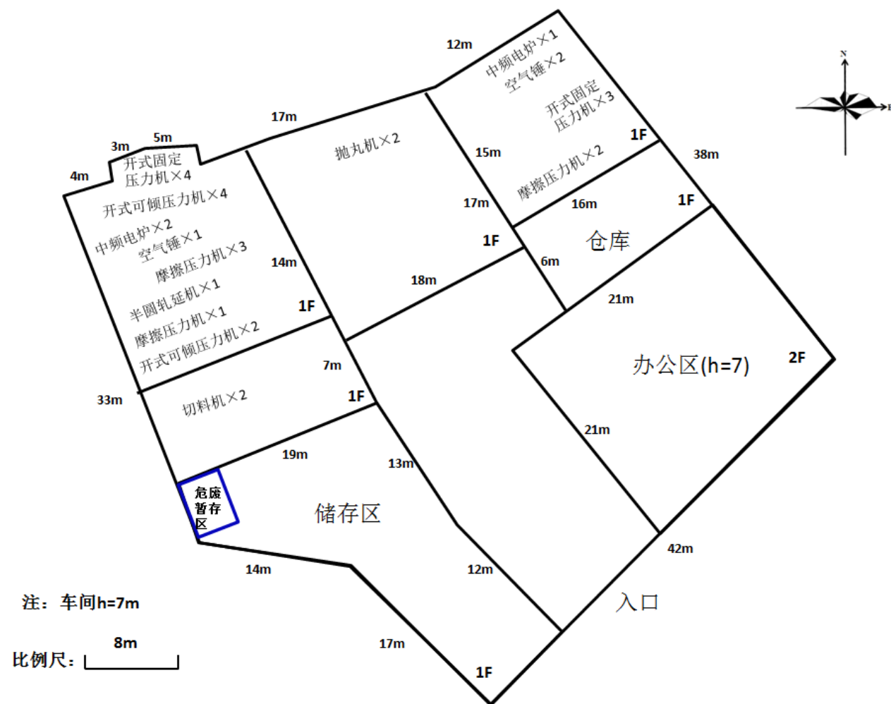
附图 4 项目平面布置图
