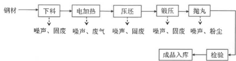
图 1-1 项目工艺流程及产污节点图
